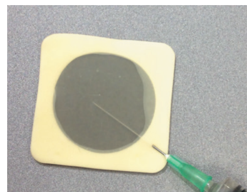
Mesure à l'aide de la méthode de Bresle visant à évaluer le niveau de concentration des sels solubles sur une surface fraîchement sablée
